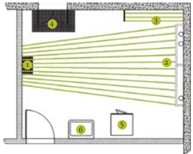
SECOMAT Wäschehänge mit Konsolen vor Leitungsrohren
