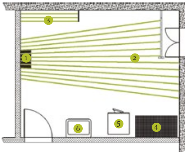
SECOMAT Wäschehänge mit Teleskop vor Fenster
